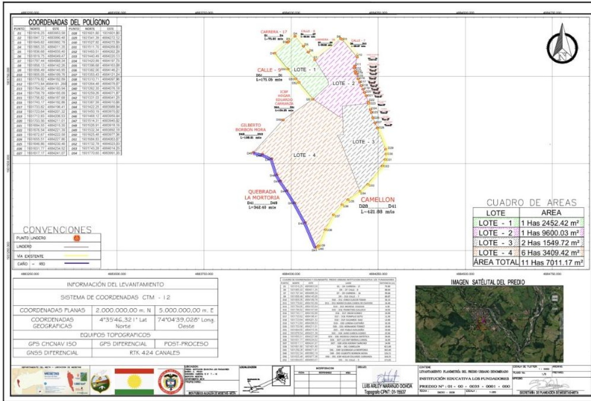
Entrega de levantamiento topográfico
